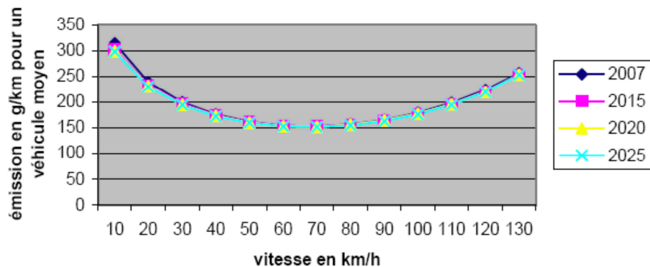
Courbes d'émissions pour les VL
