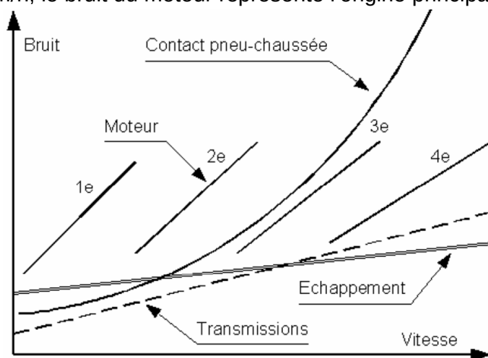
Figure 4 : Influence du revêtement de la chaussée sur les émissions sonores (Cftr (42))
