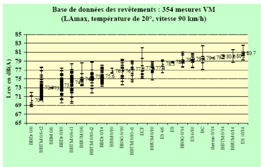
Figure 5 : Performances des revêtements (LRPC Strasbourg (43))
