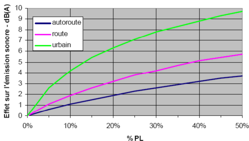
Figure 2 : Influence de la proportion de PL sur les émissions sonores (41)
