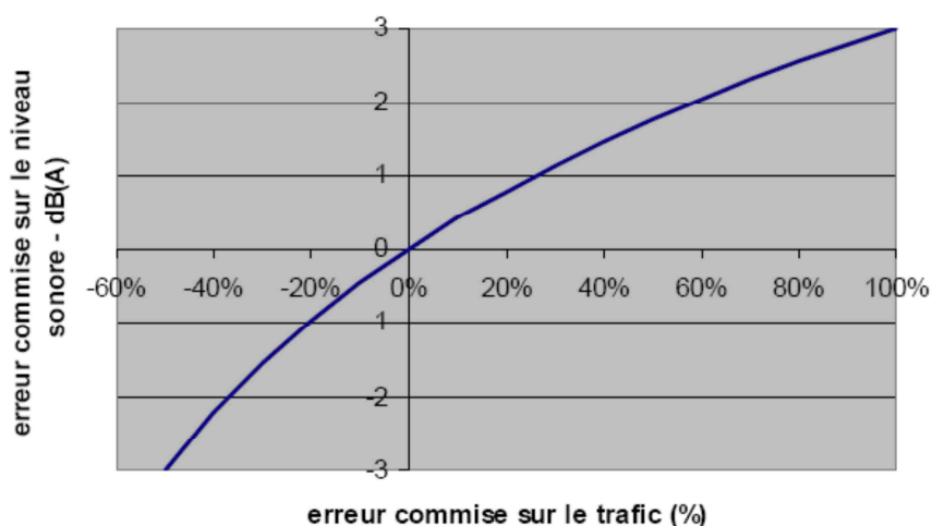
Figure 1 : Erreur commise sur le niveau sonore en fonction de l'erreur commise sur le trafic (41)
