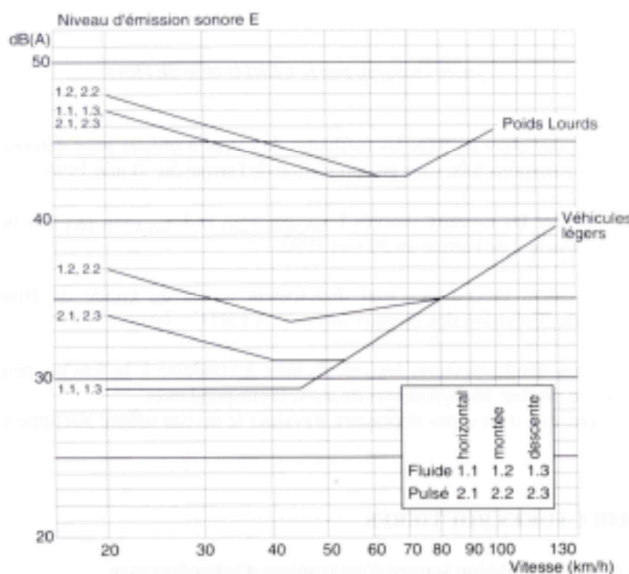
Figure 3 : Niveau d'émission sonore en fonction de la vitesse du véhicule (CETUR (28))
