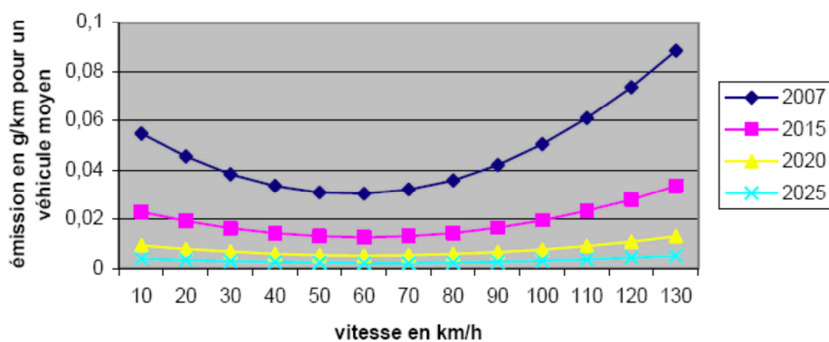
Emissions en fonction de la vitesse _ CO2 _ VL
